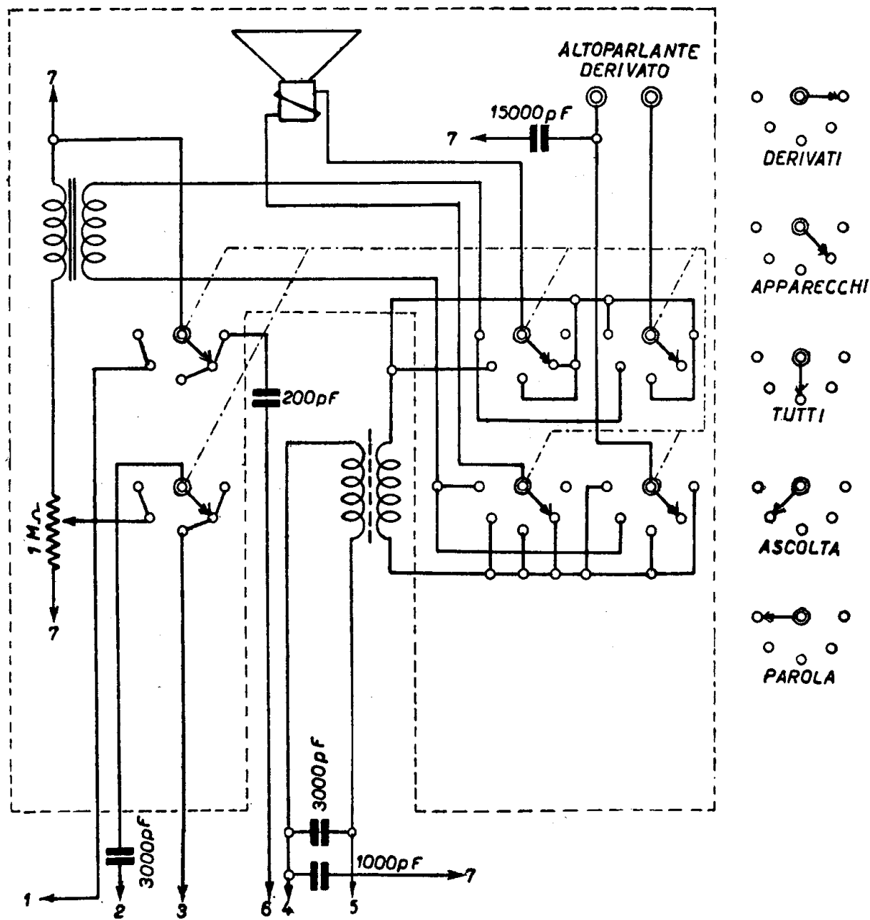
REOM - Sintomagic Radio mod. Multivox - Adatto per gli apparecchi mod. a10 e c1. Trasforma l'apparecchio radio in interfono per comunicazioni bilaterali a viva voce e riproduzione radio e fono in diversi ambienti.
